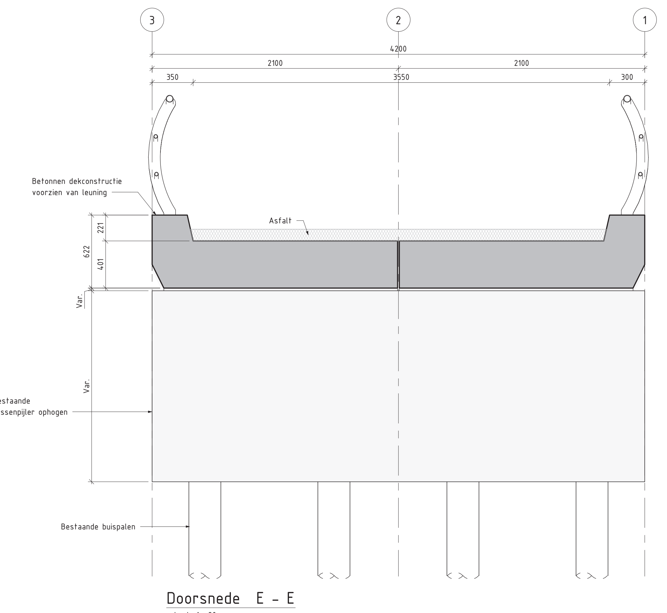
Doorsnede E - E schaal 1:20
