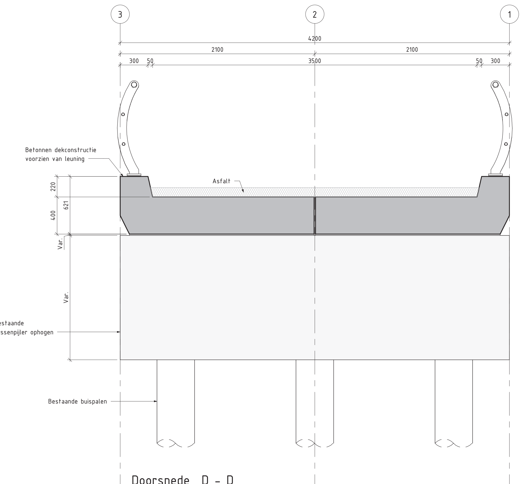
Doorsnede D - D schaal 1:20
